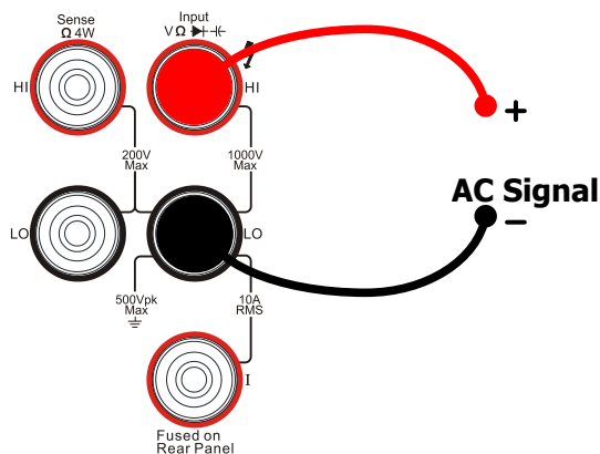
图 2-30 频率测量连接示意图
