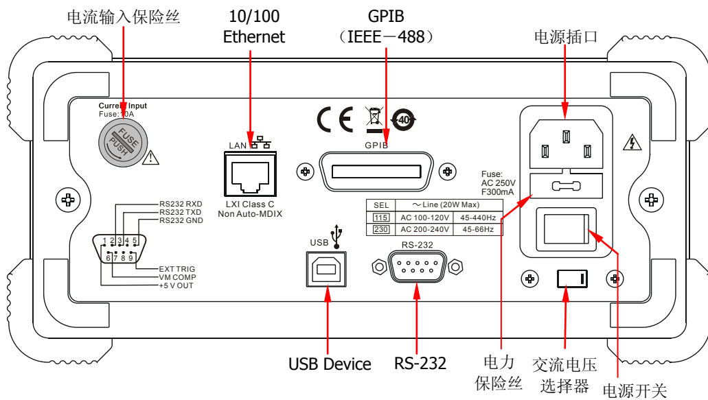
图 1-4 DM3058 后面板示意图
