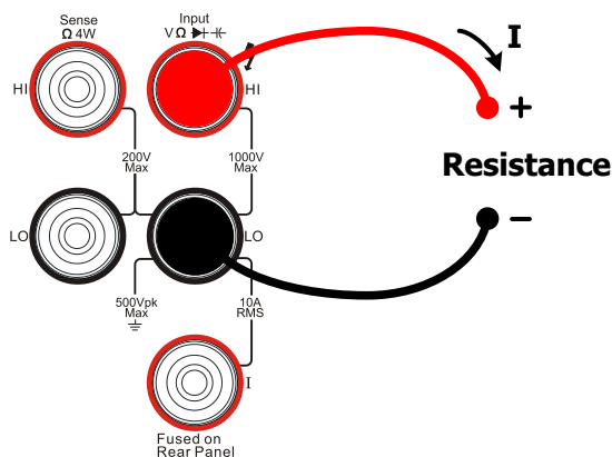
图 2-17 二线电阻测量连接示意图
