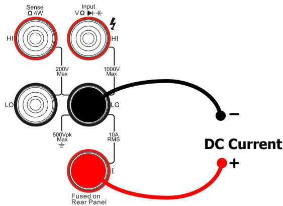
图 2-11 直流电流测量连接示意图
