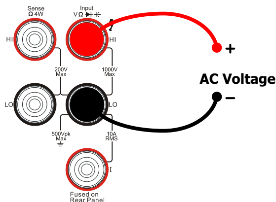
图 2-7 交流电压测量连接示意图
