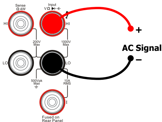
图 2-33 周期测量连接示意图
