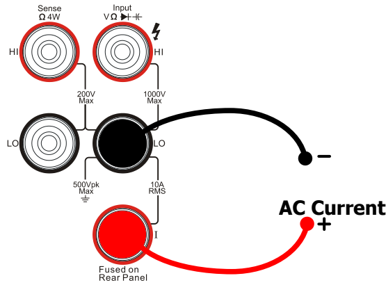
图 2-14 交流电流测量连接示意图
