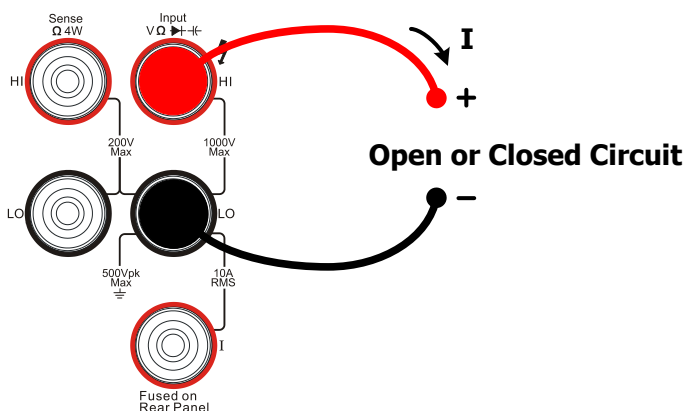
图 2-26 连通性测试示意图
