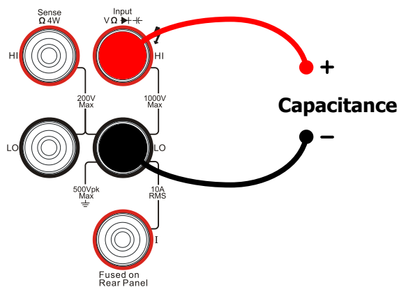
图 2-23 电容测量连接示意图
