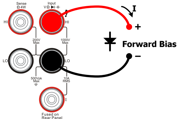
图 2-28 二极管检测示意图
