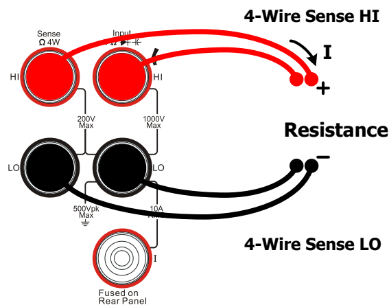
图 2-20 四线电阻测量示意图
