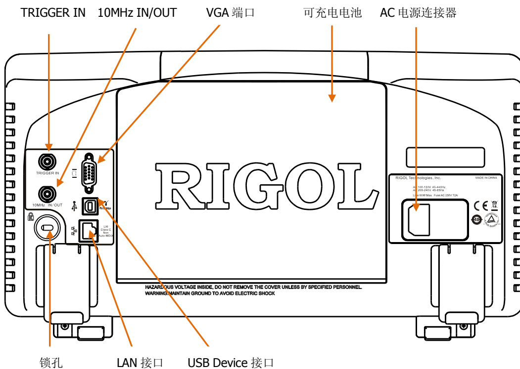
图 1-7 后面板视图
