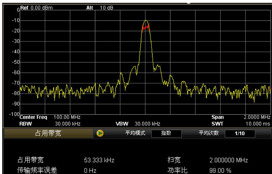
图 3-9 占用带宽测量结果
