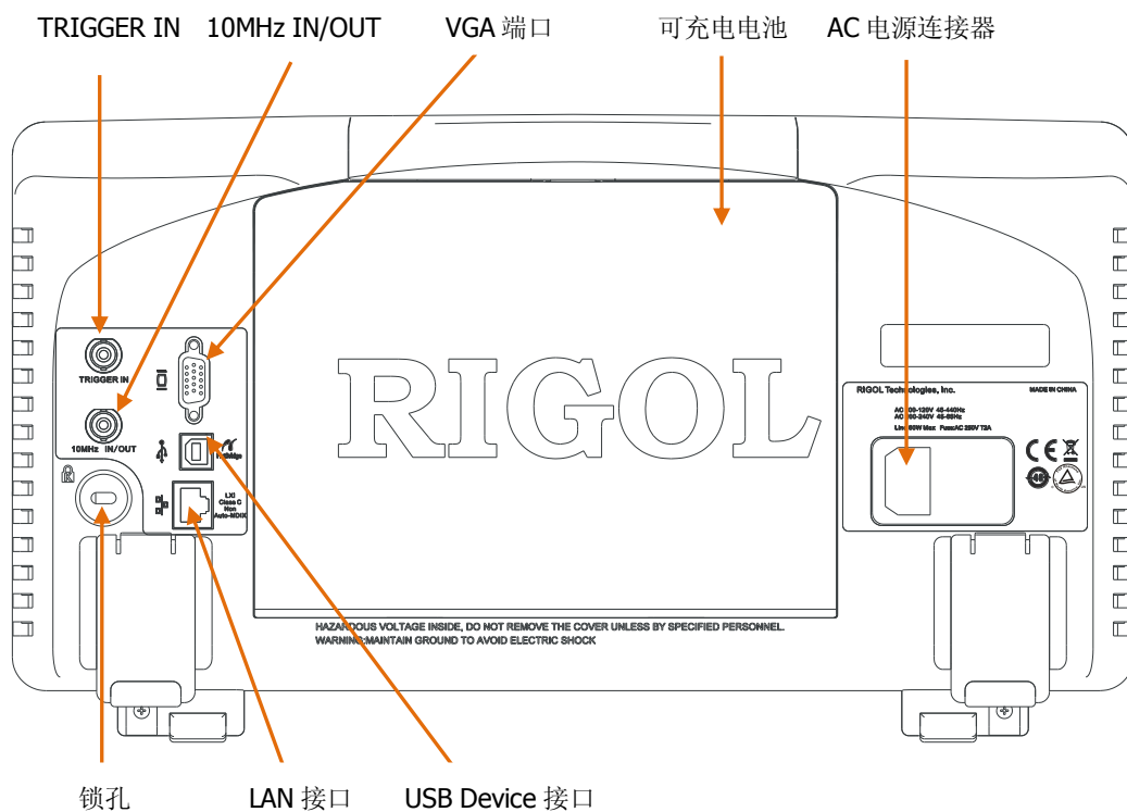
图 1-7 后面板视图
