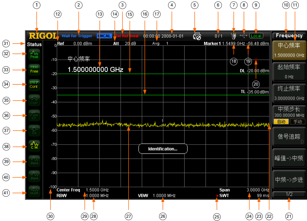
图 1-20 用户界面
