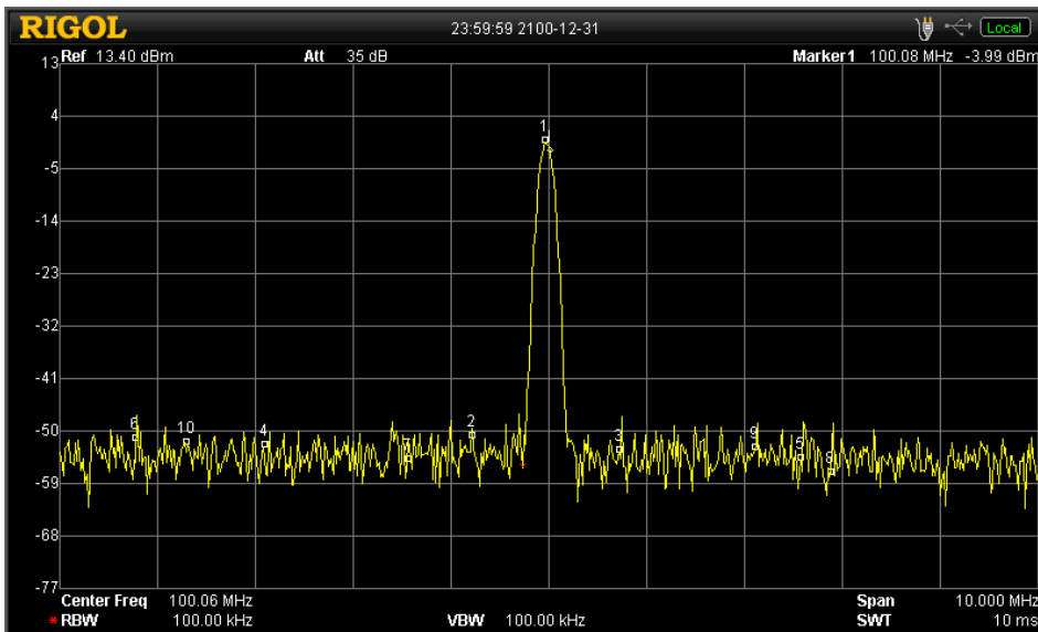
图 2-34 全屏显示
