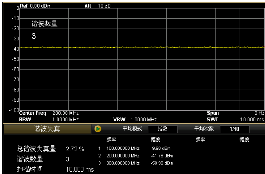
图 3-13 高级功能测量谐波失真
